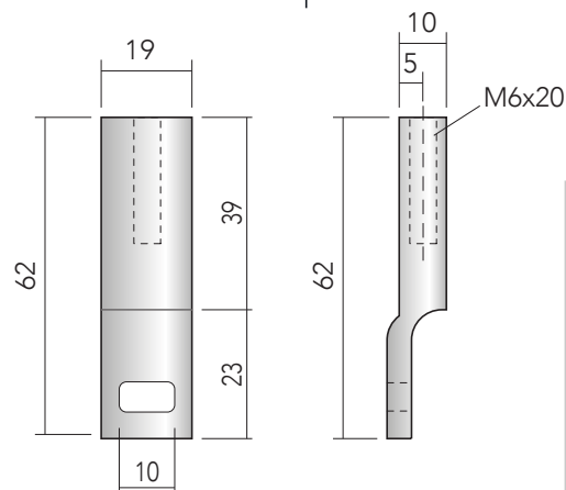
REGGITUBO CENTRALE CENTRAL BRACKET
