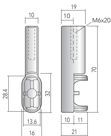
REGGITUBO LATERALE SIDE BRACKET
